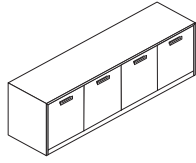
IA24/4A cm. 242x60x58 h.
